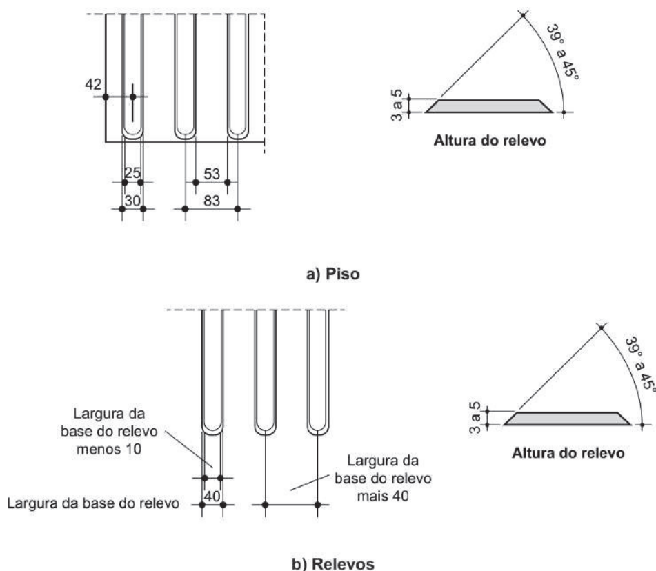
Figura 19 - Sinalização tátil direcional e relevos táteis direcionais (dimensões em milímetros)
